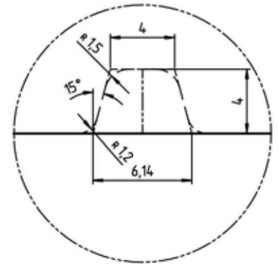
PART. TACCA / SCALA 5:1
